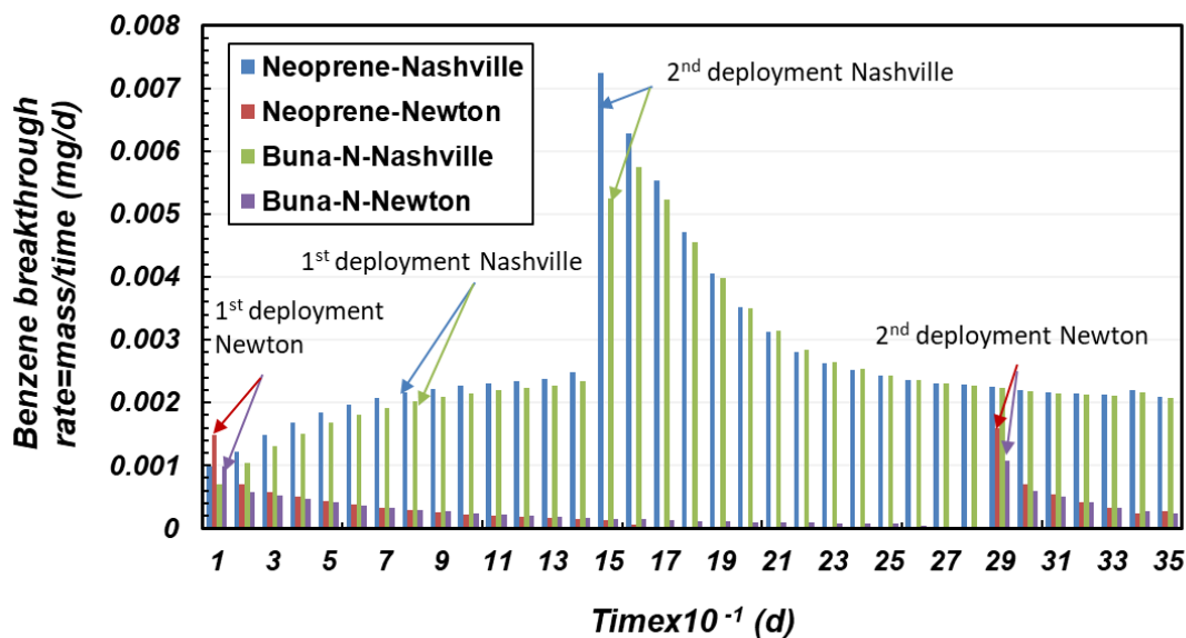
(a) Benzene
